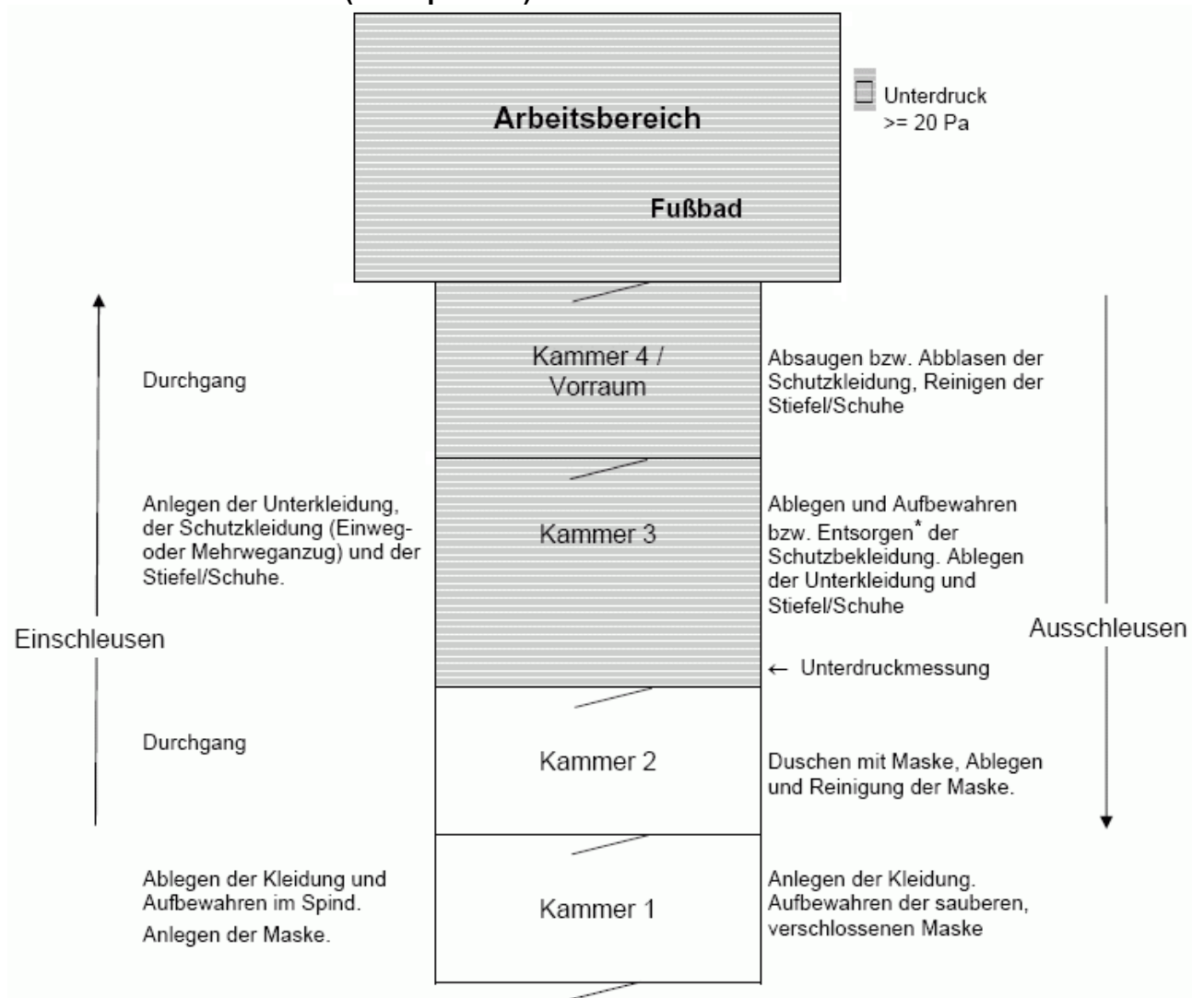
Abb. 1 Personenschleuse (Prinzipskizze)
